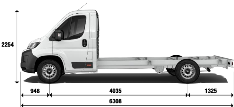
ŠASIJA S KABINO L4
