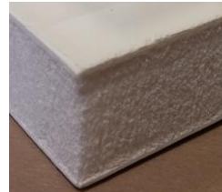
Stene Cargo Box - Poliestrska plošča iz steklenih vlaken z gelcoat premazom, lahka in trpežna zasnova za večjo nosilnost vozila
