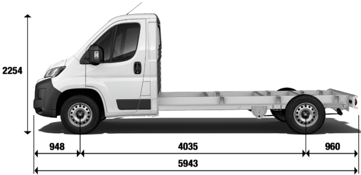
ŠASIJA S KABINO L3
