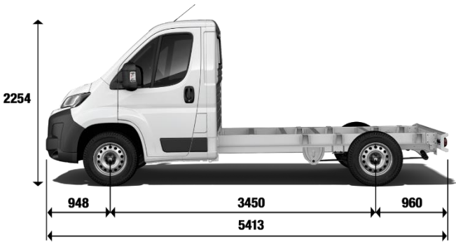
ŠASIJA S KABINO L2
