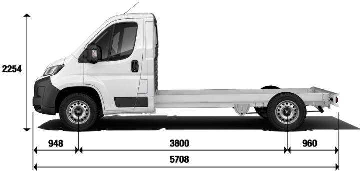
ŠASIJA S KABINO L2+
