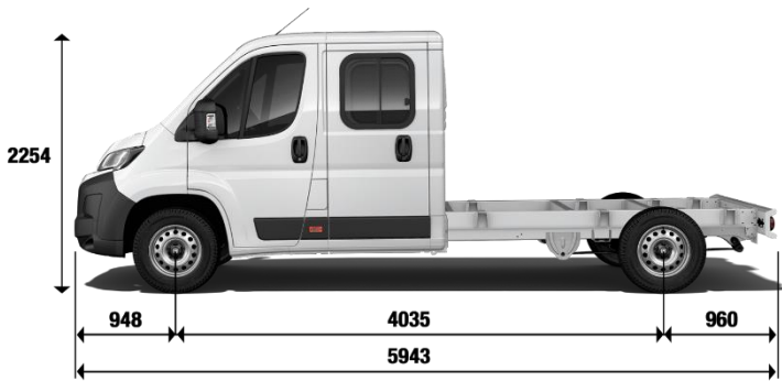
ŠASIJA Z DVOJNO KABINO L3
